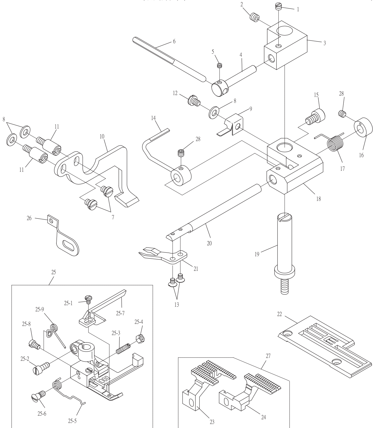
25. 壓腳編號列表 Press Foot
